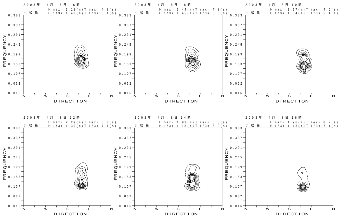
図 - 13.44 小松島 代表的な高波期間中の方向スペクトル
