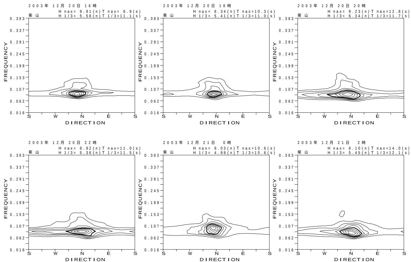
図 - 13.12 柴山 代表的な高波期間中の方向スペクトル
