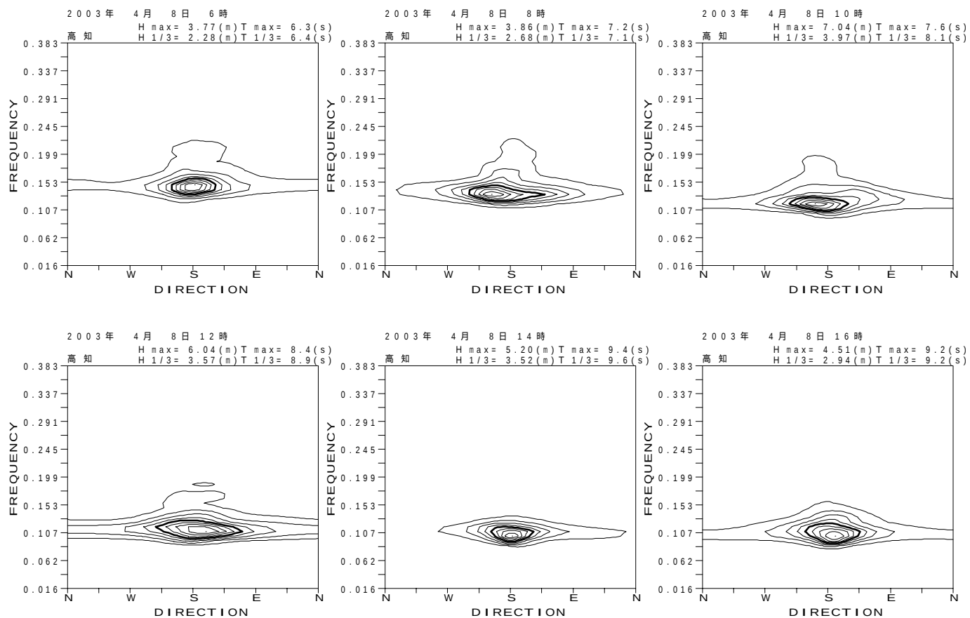
図 - 13.46 高知 代表的な高波期間中の方向スペクトル
