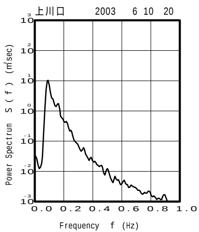
図 - 13.47 上川口 代表的な高波期間中のスペクトル
