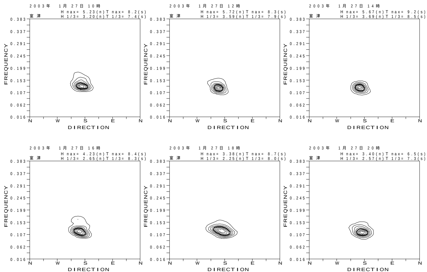
図 - 13.45 室津 代表的な高波期間中の方向スペクトル
