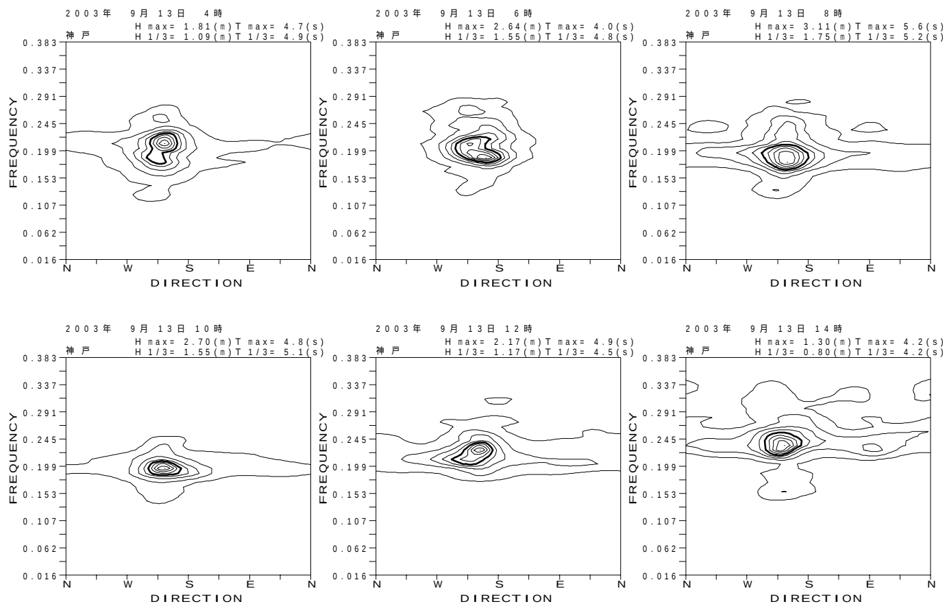
図 - 13.43 神戸 代表的な高波期間中の方向スペクトル
