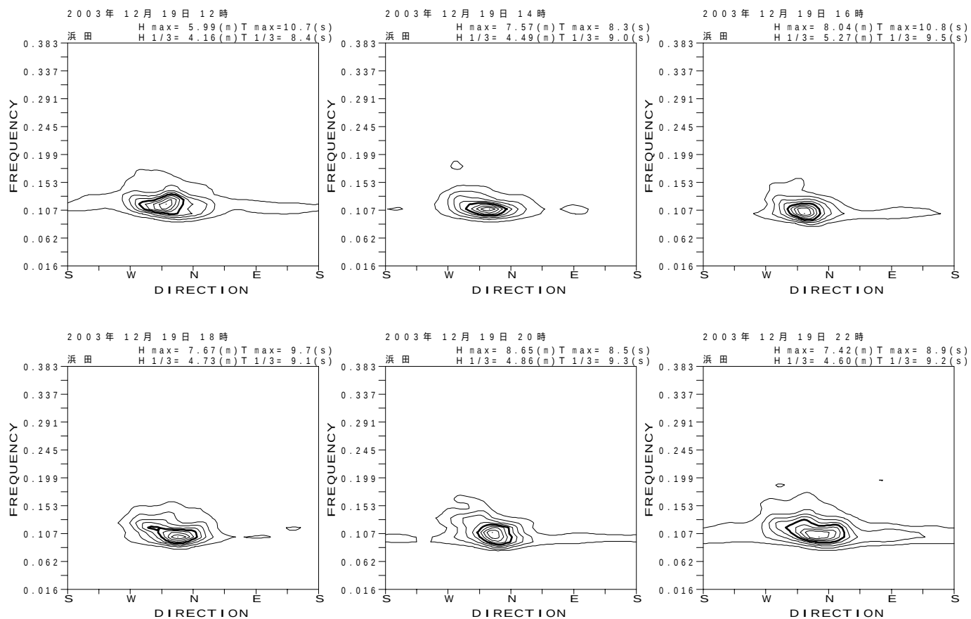
図 - 13.16 浜田 代表的な高波期間中の方向スペクトル
