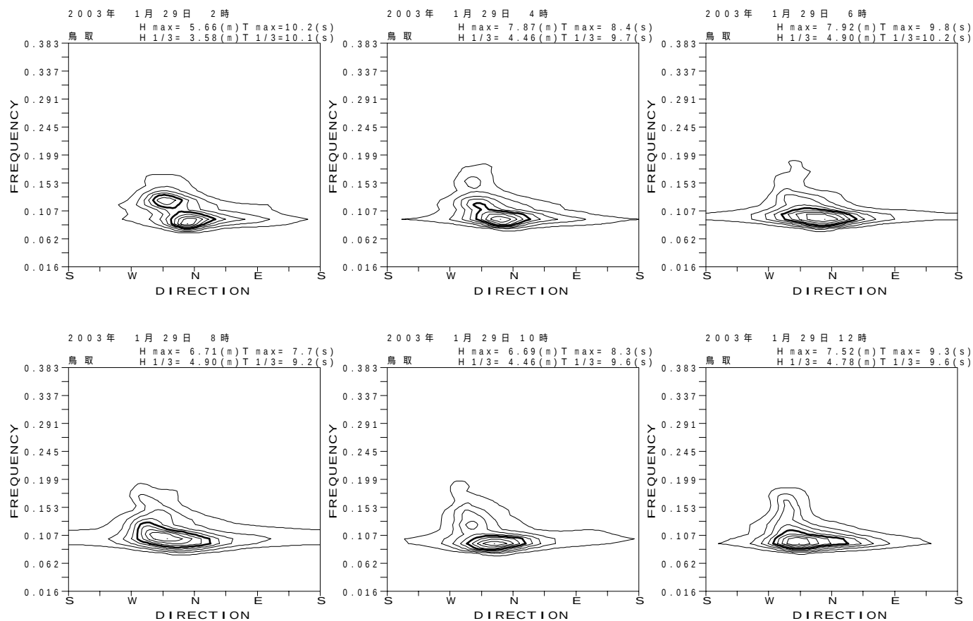
図 - 13.14 鳥取 代表的な高波期間中の方向スペクトル
