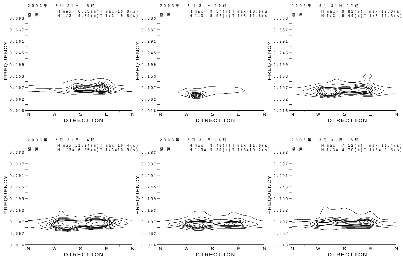
図 - 13.42 潮 岬 代表的な高波期間中の方向スペクトル
