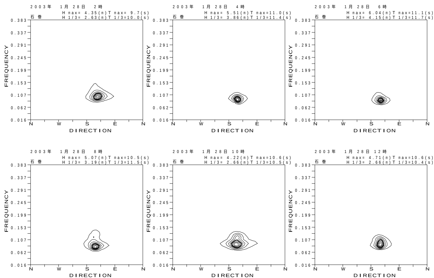
図 - 13.29 石巻 代表的な高波期間中の方向スペクトル
