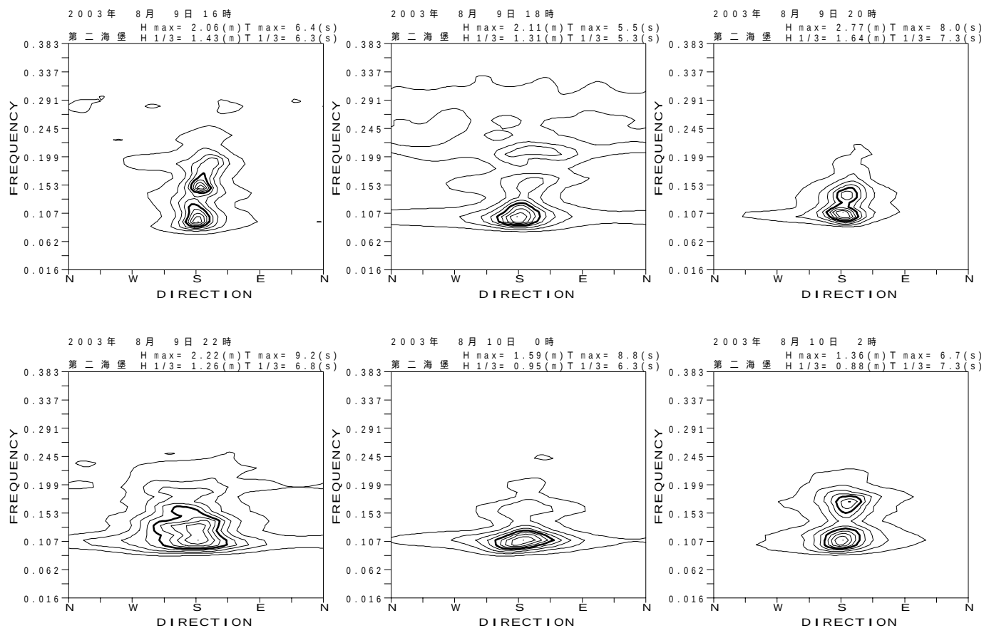
図 - 13.35 第二海堡 代表的な高波期間中の方向スペクトル
