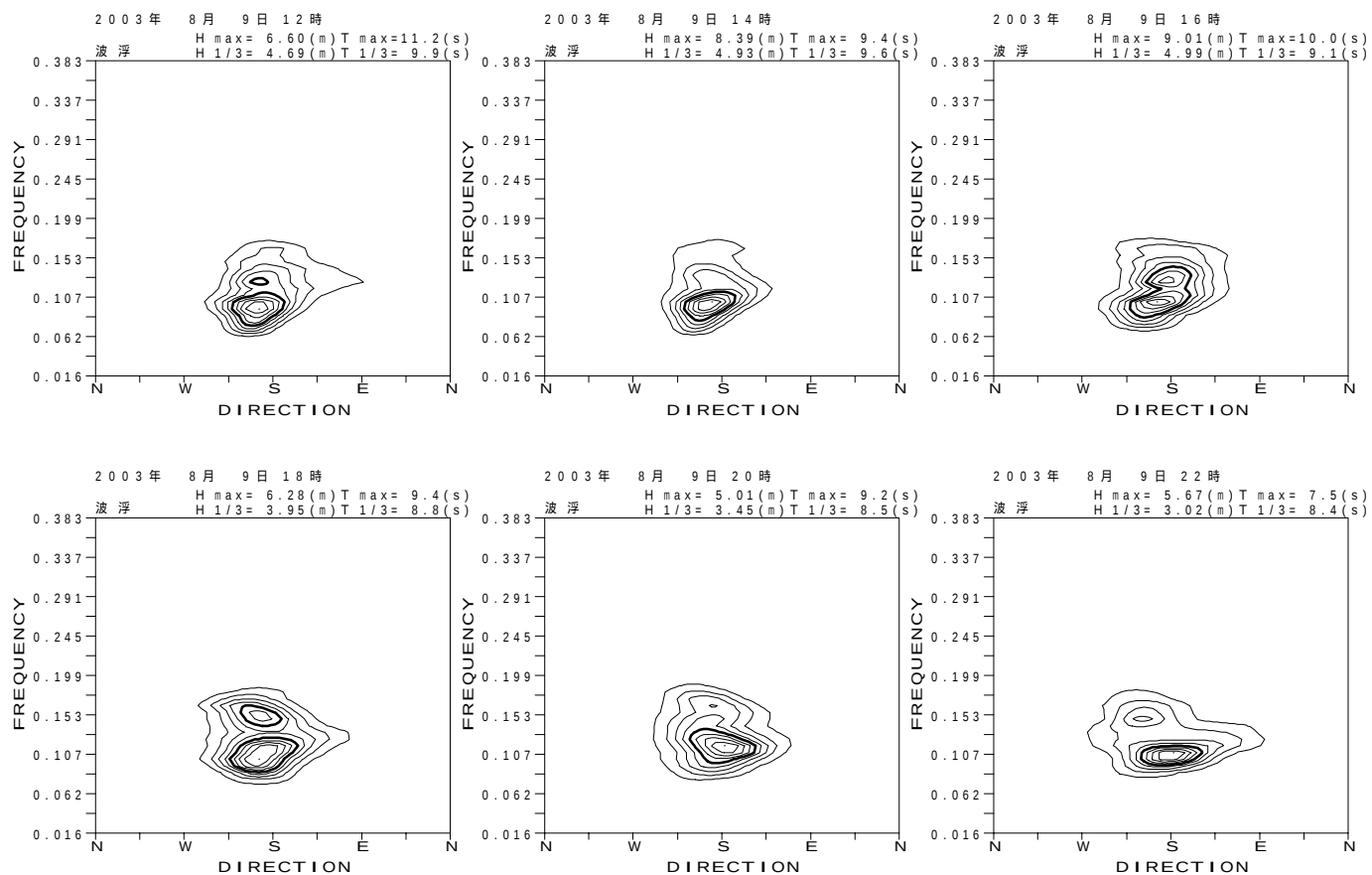
図 - 13.37 波浮 代表的な高波期間中の方向スペクトル
