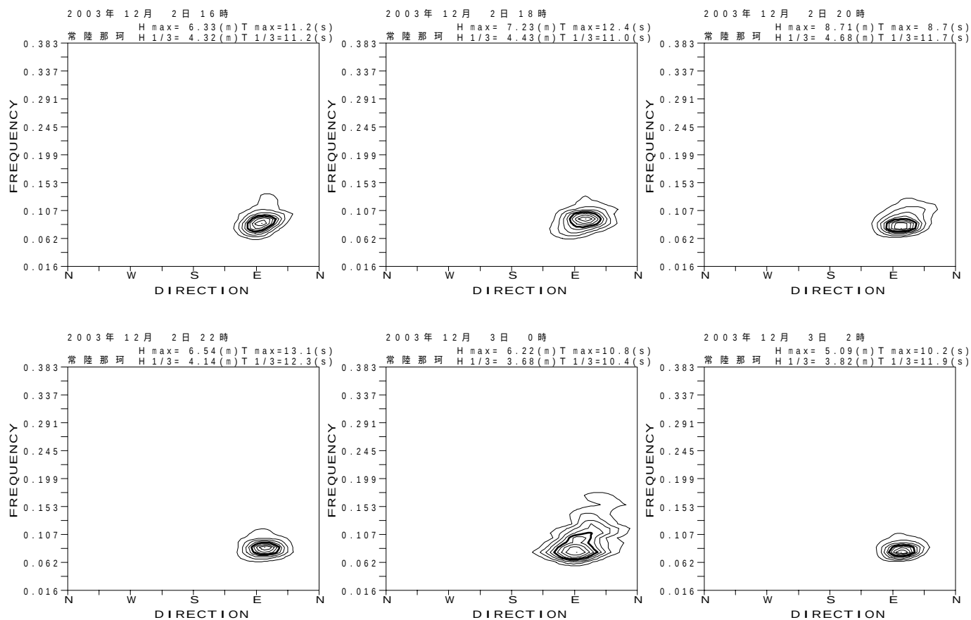
図 - 13.33 常陸那珂 代表的な高波期間中の方向スペクトル
