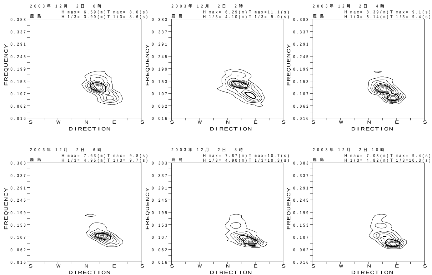
図 - 13.34 鹿島 代表的な高波期間中の方向スペクトル
