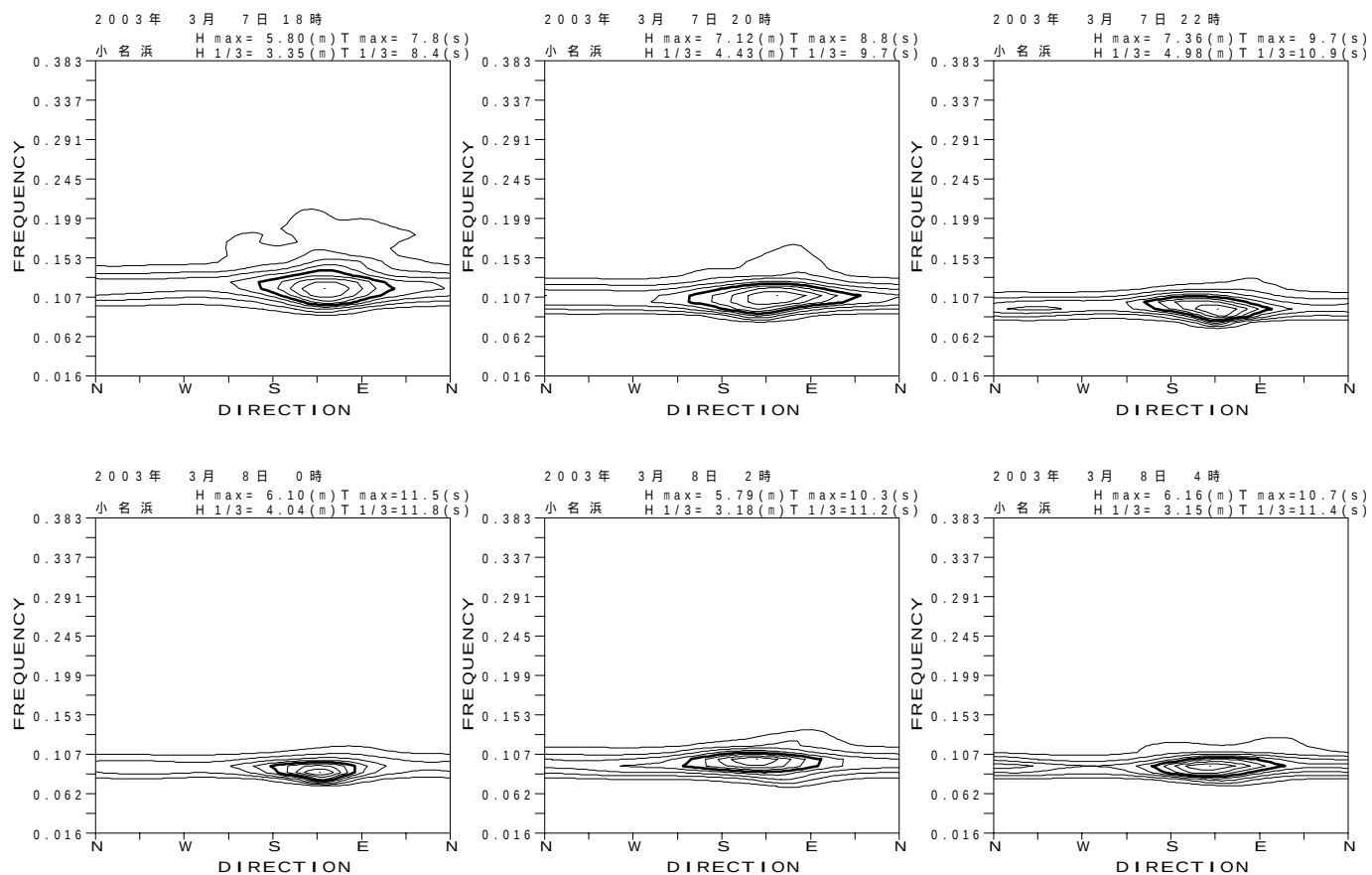
図 - 13.32 小名浜 代表的な高波期間中の方向スペクトル
