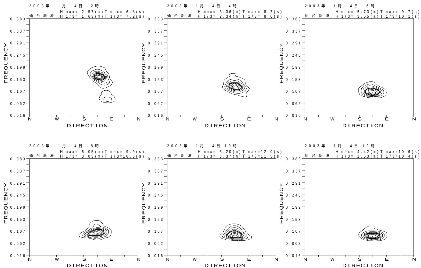
図 - 13.30 仙台新港 代表的な高波期間中の方向スペクトル
