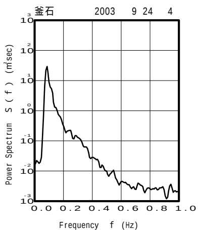
図 - 13.28 釜石 代表的な高波期間中のスペクトル
