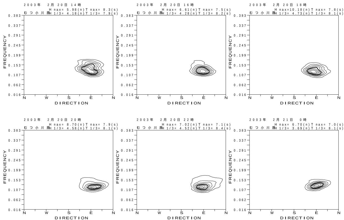
図 - 13.25 むつ小川原 代表的な高波期間中の方向スペクトル
