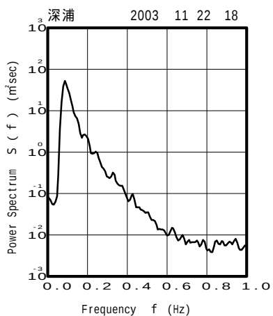
図 - 13.3 深浦 代表的な高波期間中のスペクトル
