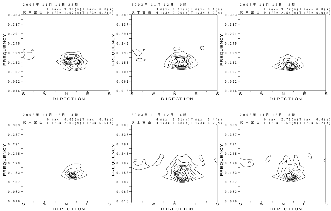
図 - 13.9 伏木富山 代表的な高波期間中の方向スペクトル
