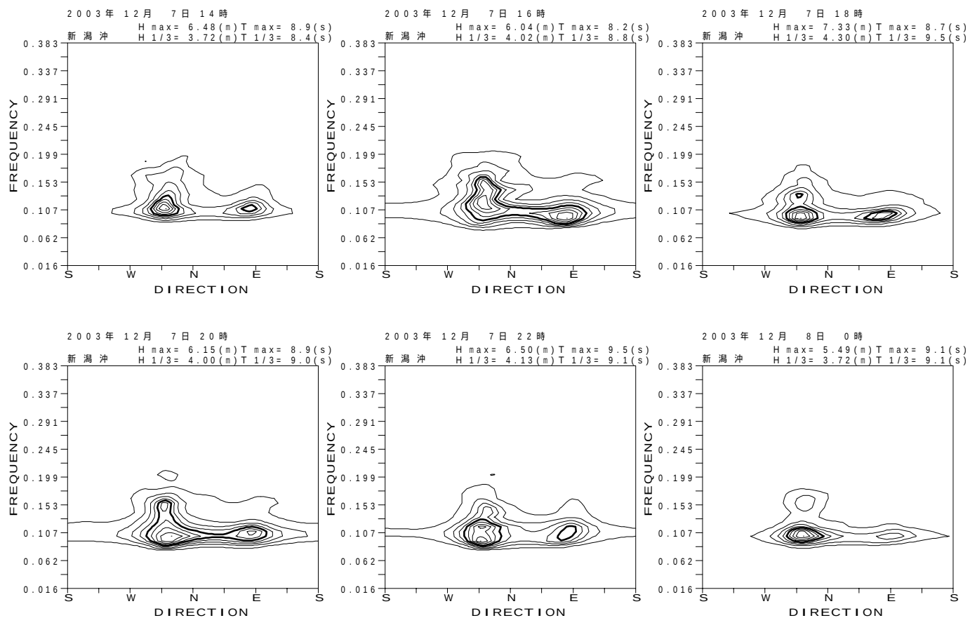
図 - 13.6 新潟沖 代表的な高波期間中の方向スペクトル
