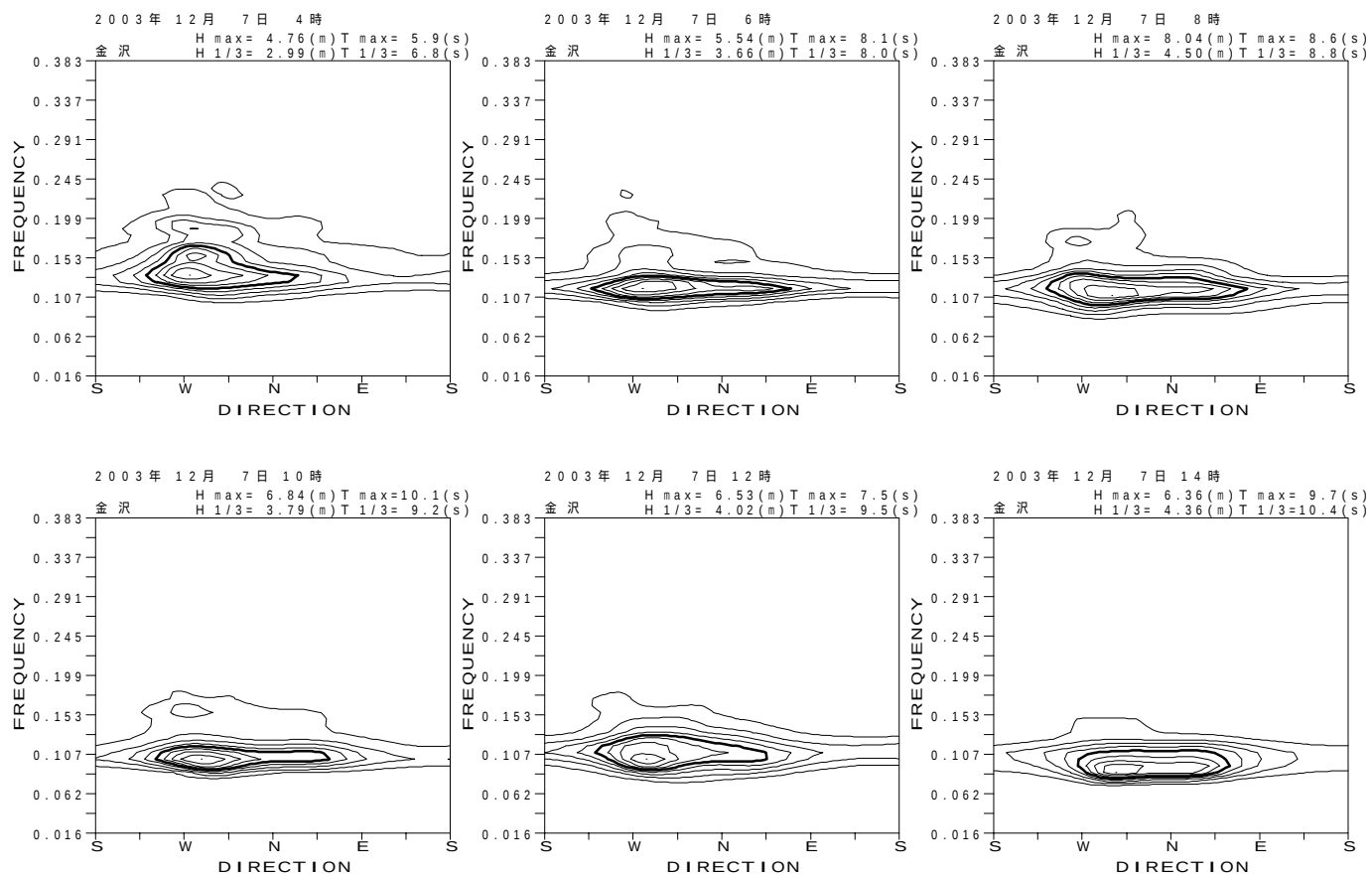
図 - 13.11 金沢 代表的な高波期間中の方向スペクトル
