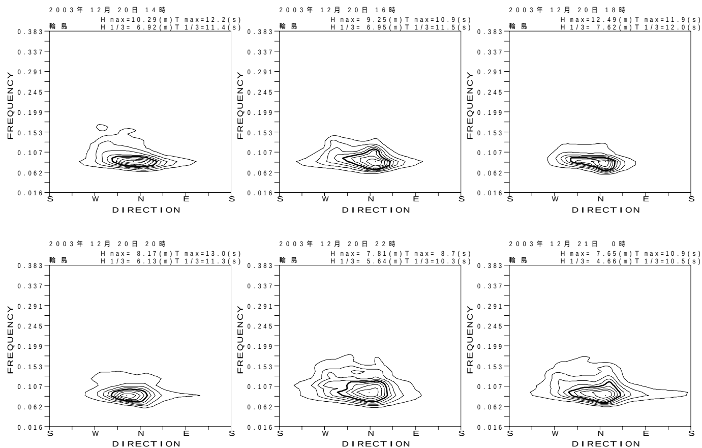
図 - 13.10 輪島 代表的な高波期間中の方向スペクトル
