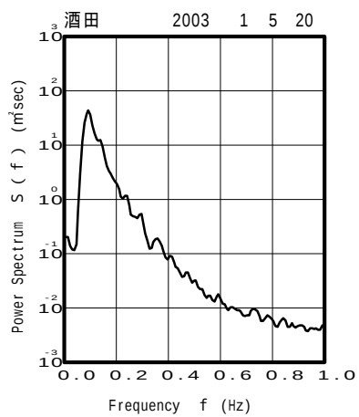
図 - 13.5 酒田 代表的な高波期間中のスペクトル
