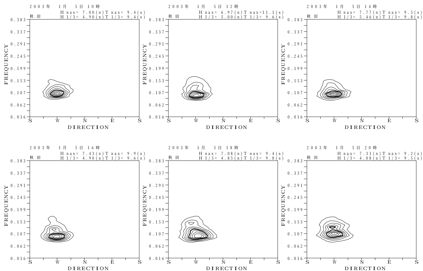
図-13.4 秋田 代表的な高波期間中の方向スペクトル
