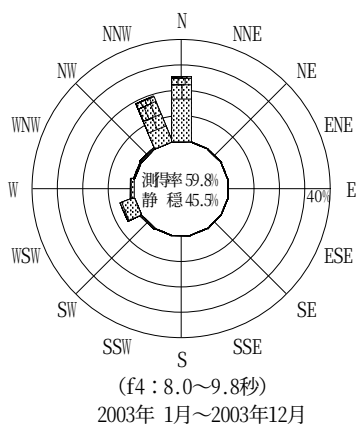
図-12.21 那覇 波高・波向別出現頻度図 (f2, f3, f4, f5, 全周期帯)
