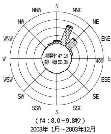
図 - 12.22 紋別(南) 波高・波向別出現頻度図 ( f2 , f3 , f4 , f5 , 全周期帯 )
