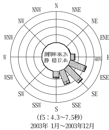
図-12.23 十勝 波高・波向別出現頻度図 (f2, f3, f4, f5, 全周期帯)
