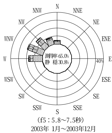
図-12.1 留萌 波高・波向別出現頻度図 (f2, f3, f4, f5, 全周期帯)
