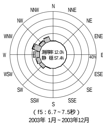
図 - 12.2 瀬棚 波高・波向別出現頻度図 ( f2 , f3 , f4 , f5 , 全周期帯 )
