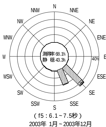
図 - 12.24 苦小牧 波高・波向別出現頻度図 ( f2 , f3 , f4 , f5 , 全周期帯 )
