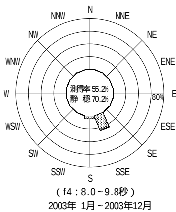
図 - 12.39 清水 波高・波向別出現頻度図 ( f2 , f3 , f4 , f5 , 全周期帯 )
