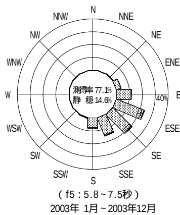
図 - 12.49 細島 波高・波向別出現頻度図 ( f2 , f3 , f4 , f5 , 全周期帯 )
