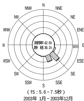
図 - 12.51 志布志湾 波高・波向別出現頻度図 ( f2 , f3 , f4 , f5 , 全周期帯 )
