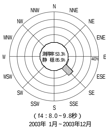
図 - 12.44 小松島 波高・波向別出現頻度図 ( f2 , f3 , f4 , f5 , 全周期帯 )
