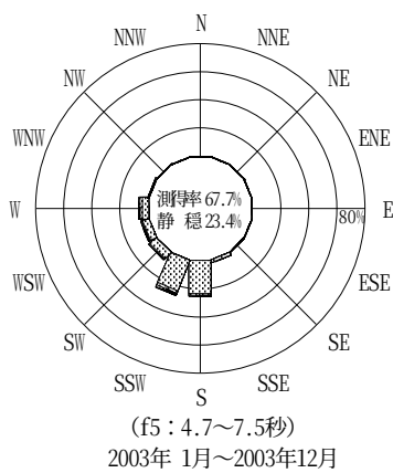
図-12.45 室津 波高・波向別出現頻度図 (f2, f3, f4, f5, 全周期帯)
