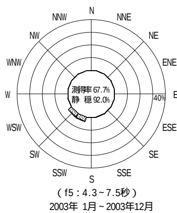
図 - 12.43 神戸 波高・波向別出現頻度図 ( f2 , f3 , f4 , f5 , 全周期帯 )
