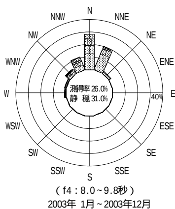
図 - 12.16 浜田 波高・波向別出現頻度図 ( f2 , f3 , f4 , f5 , 全周期帯 )
