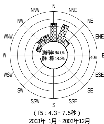
図 - 12.14 鳥取 波高・波向別出現頻度図 ( f2 , f3 , f4 , f5 , 全周期帯 )
