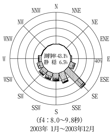
図-12.42 潮岬 波高・波向別出現頻度図 (f2, f3, f4, f5, 全周期帯)
