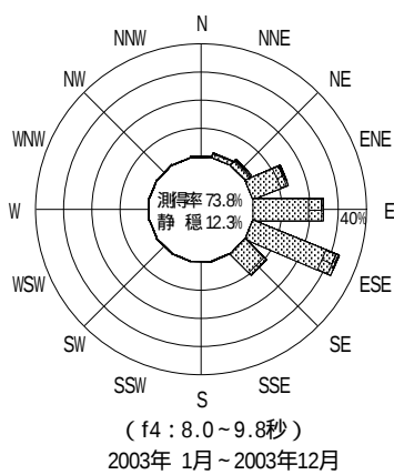
図 - 12.27 久慈 波高・波向別出現頻度図 ( f2 , f3 , f4 , f5 , 全周期帯 )
