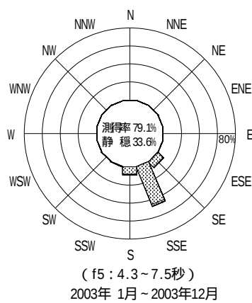
図 - 12.29 石巻 波高・波向別出現頻度図 ( f2 , f3 , f4 , f5 , 全周期帯 )
