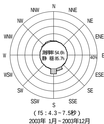
図 - 12.35 第二海堡 波高・波向別出現頻度図 ( f2 , f3 , f4 , f5 , 全周期帯 )
