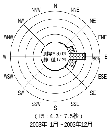
図 - 12.31 相馬 波高・波向別出現頻度図 ( f2 , f3 , f4 , f5 , 全周期帯 )
