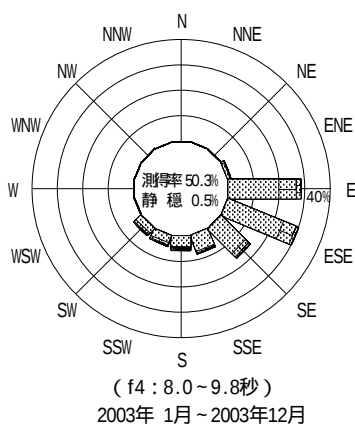
図 - 12.37 波浮 波高・波向別出現頻度図 ( f2 , f3 , f4 , f5 , 全周期帯 )
