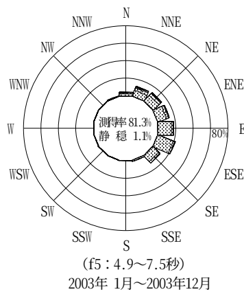
図-12.33 常陸那珂 波高・波向別出現頻度図 (f2, f3, f4, f5, 全周期帯)
