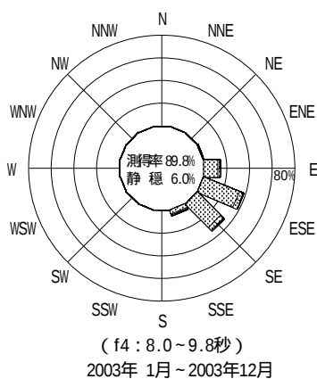
図 - 12.32 小名浜 波高・波向別出現頻度図 ( f2 , f3 , f4 , f5 , 全周期帯 )
