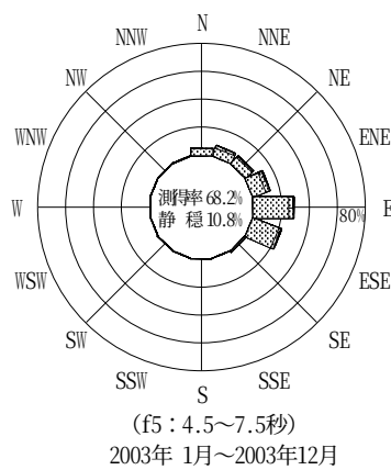
図-12.26 八戸 波高・波向別出現頻度図 (f2, f3, f4, f5, 全周期帯)
