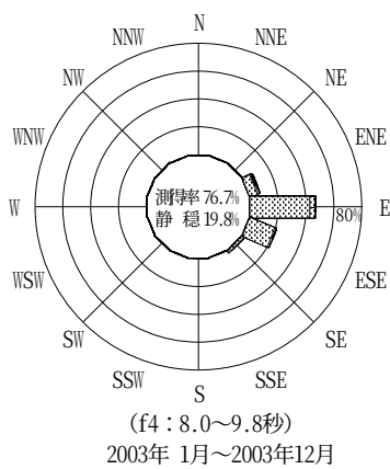
図-12.25 むつ小川原 波高・波向別出現頻度図 (f2, f3, f4, f5, 全周期帯)
