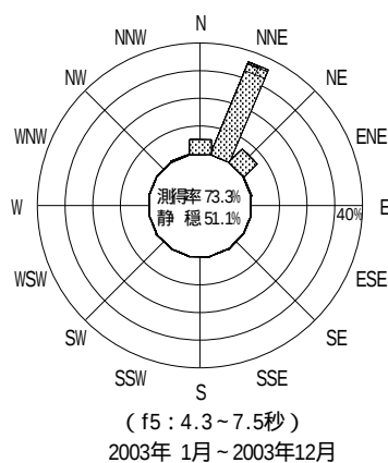
図 - 12.8 富山 波高・波向別出現頻度図 ( f2 , f3 , f4 , f5 , 全周期帯 )
